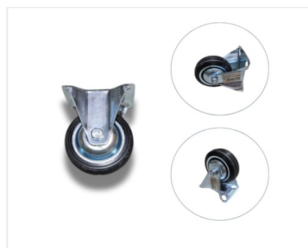
Šifra: 3502 TOČKIČ FI 100 CRNI FIKSNI 6.0 KM
