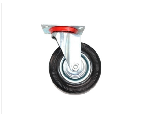
Šifra: 3505 TOČKIČ FI 125 CRNI OKRETNI 7.5 KM
